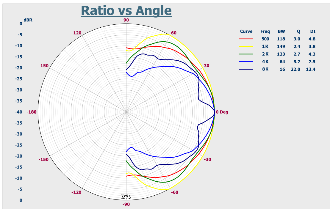
Круговая диаграмма направленности громкоговорителя LPA-6C (с клеммой на 0.75 Вт)
